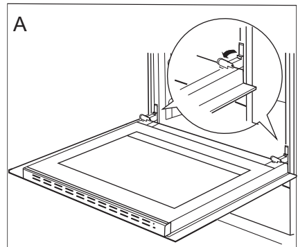
Déplacement des protections des charnières
